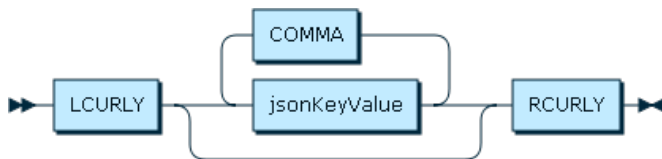
Figure 12.17 jsonDoc
